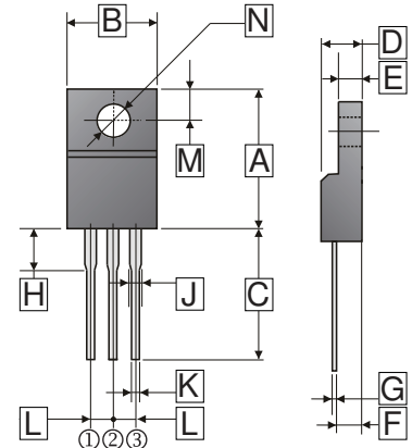
ITO-220
