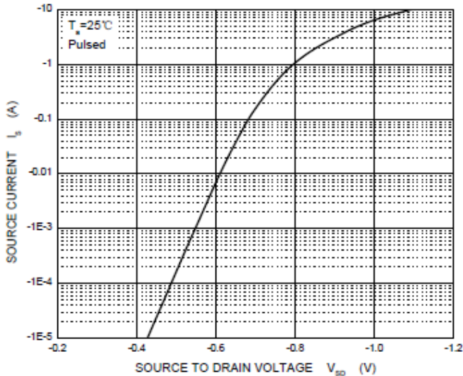
I_S — V_{SD}
