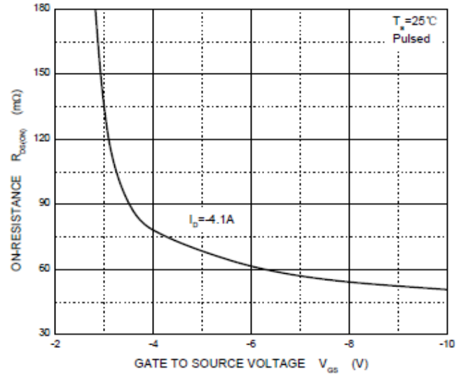
R_{DS(ON)} — V_{GS}
