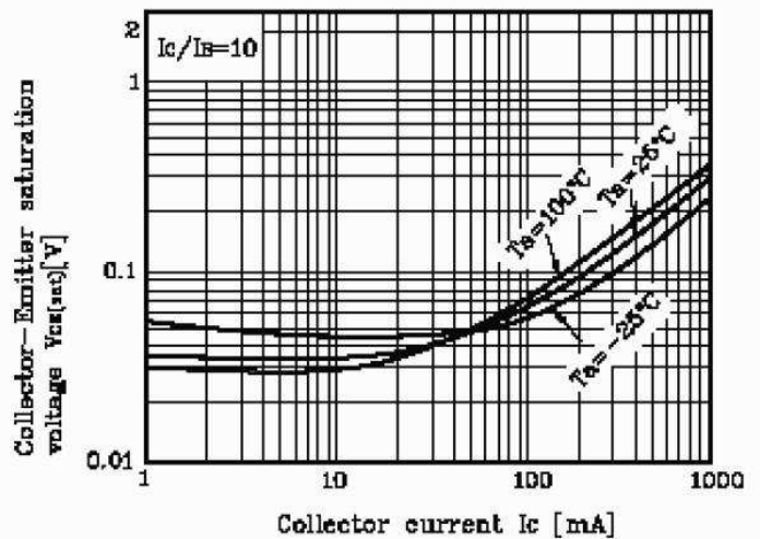
Fig. 4 V_{CE(sat)} - I_C
