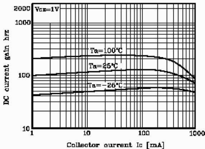
Fig. 5 h_{FE} - I_C
